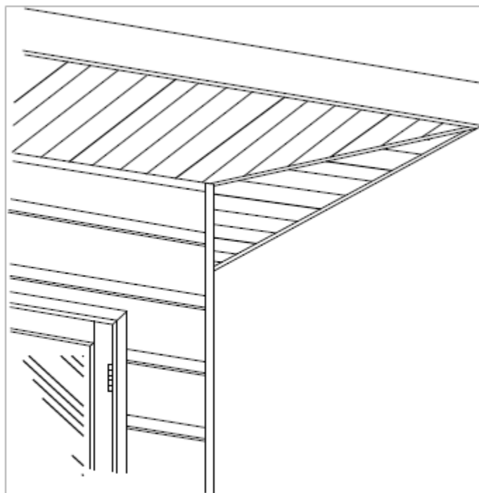
Fig 20a Soffit Detail
